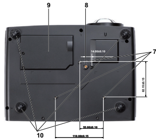
底面図
